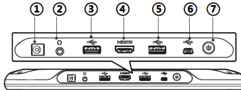
Figure 2-3 D1 Pro Tablet, Top View
